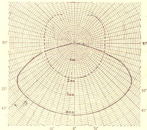
II. - Courbe des intensités lumineuses
